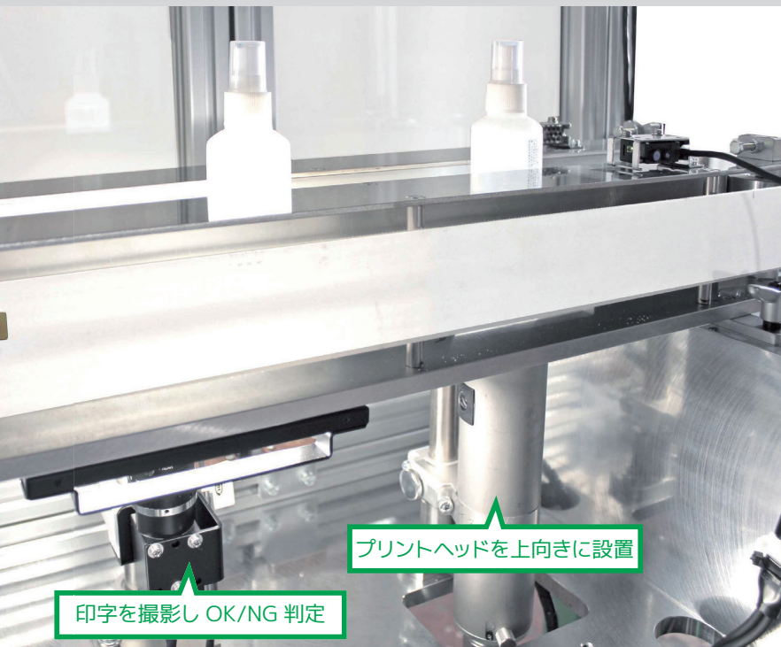
ボトル底面印字検査装置 (連続式インクジェットプリンター CCS3500+ 印字検査装置 PK100) NEW
