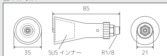
■本体寸法
