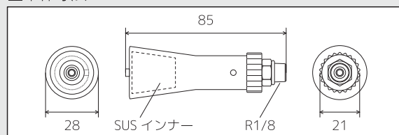
■本体寸法
