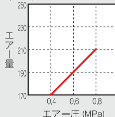
(ℓ/min) 使用エア量グラフ
