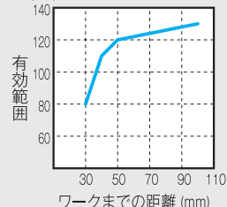
(mm) エア有効範囲グラフ
