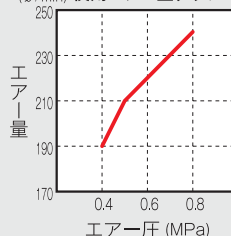
(ℓ/min) 使用エア量グラフ
